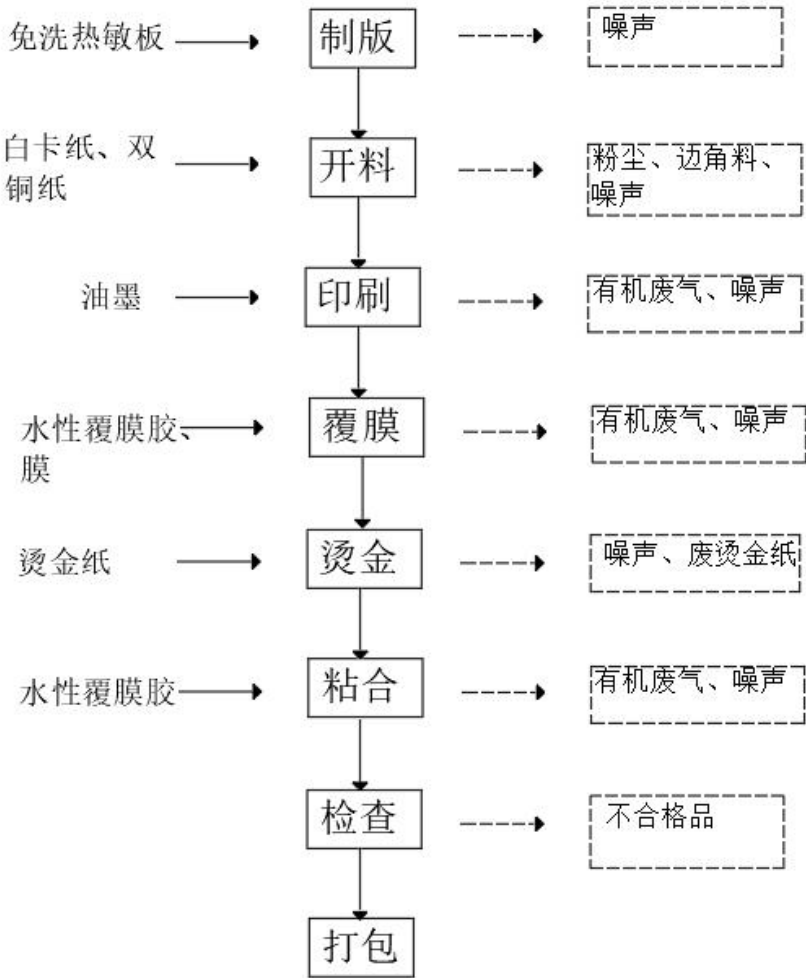
图 2-3 包装纸盒②生产工艺流程图
